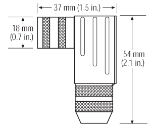
配对 D7 母接头 (90° 转弯出线) 型号: 560779 (STC09131-7)
